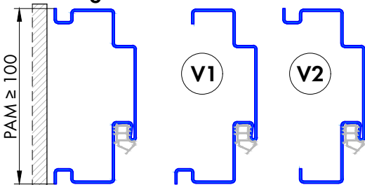
Profil 116.3
