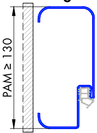
Profil 143.3
