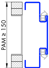
Profil 211.3
