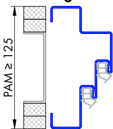
Profil 212.3
