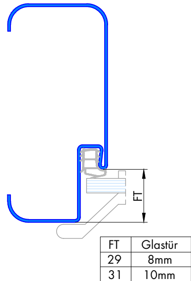
Profil 243b für stumpfes 40mm Holztürblatt
