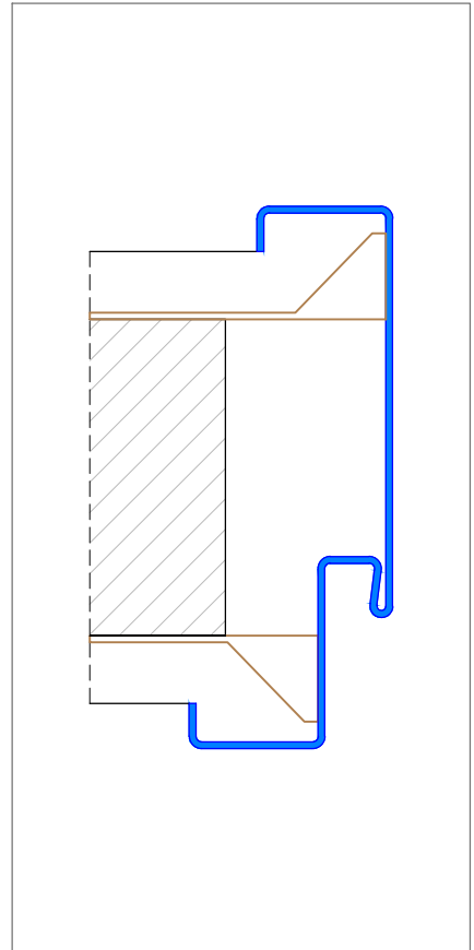
Doppelanker
