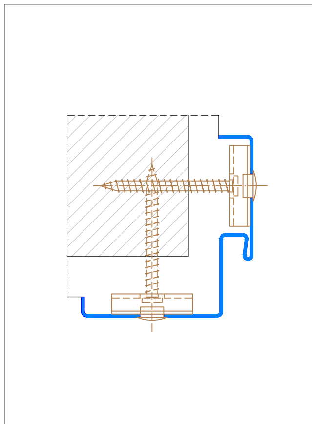
Hutanker mit Bohrung
