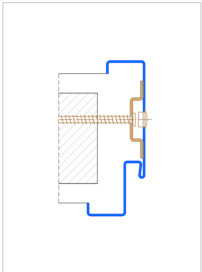
Hutanker mit Bohrung
