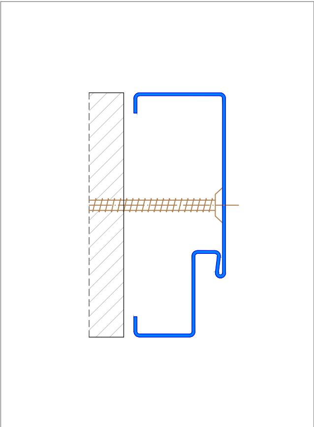
Durchzug in der Leibung
