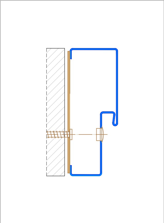
Flacheisen mit Bohrung im Falz (für stumpfe Türen)
