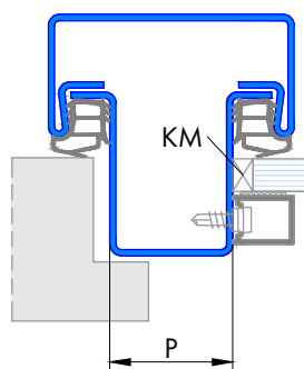
Schnitt B-B
