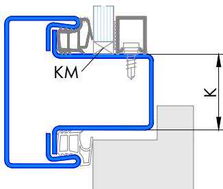
Schnitt A-A
