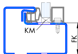
Schnitt C-C
