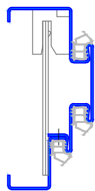
Profil 308.6
