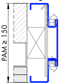
Profil 308.3
