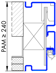
Profil 329.3
