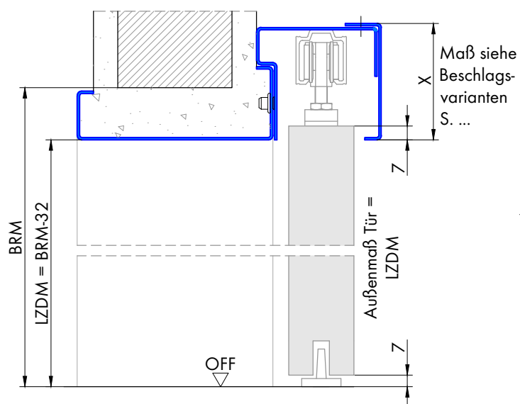
Schnitt B-B
