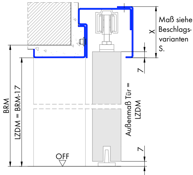
Schnitt B-B
