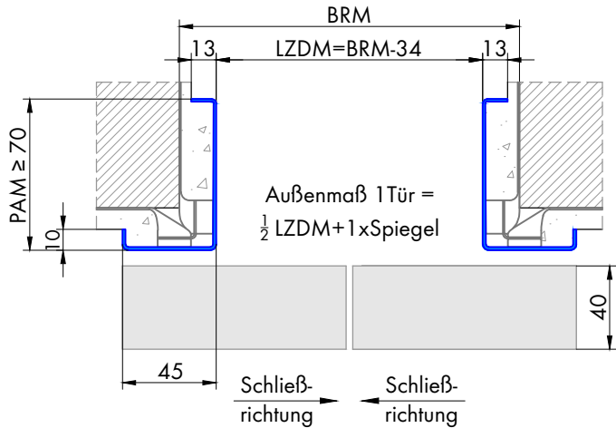
Schnitt A-A
