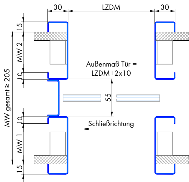
Schnitt B-B
