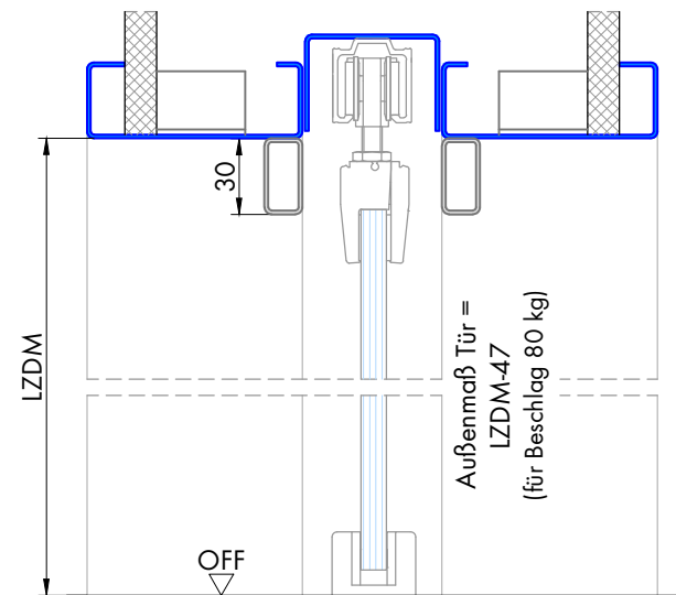
Schnitt B-B
