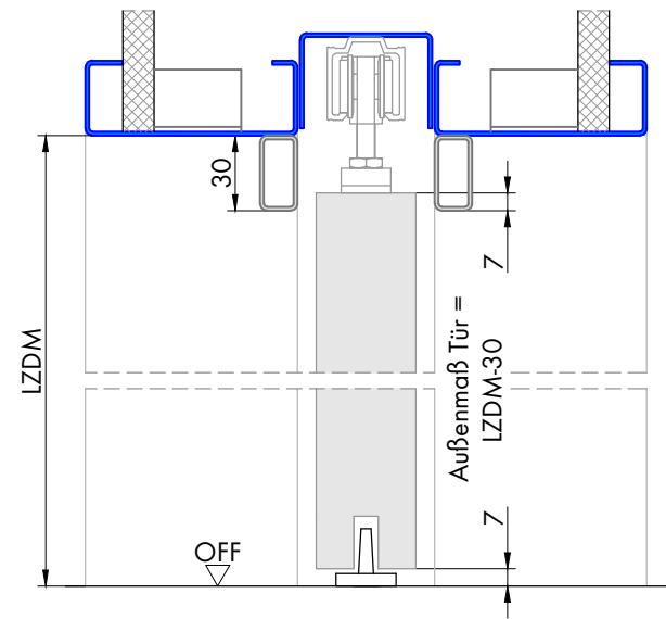
Schnitt B-B
