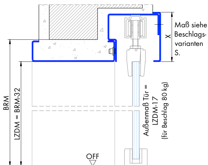
Schnitt B-B
