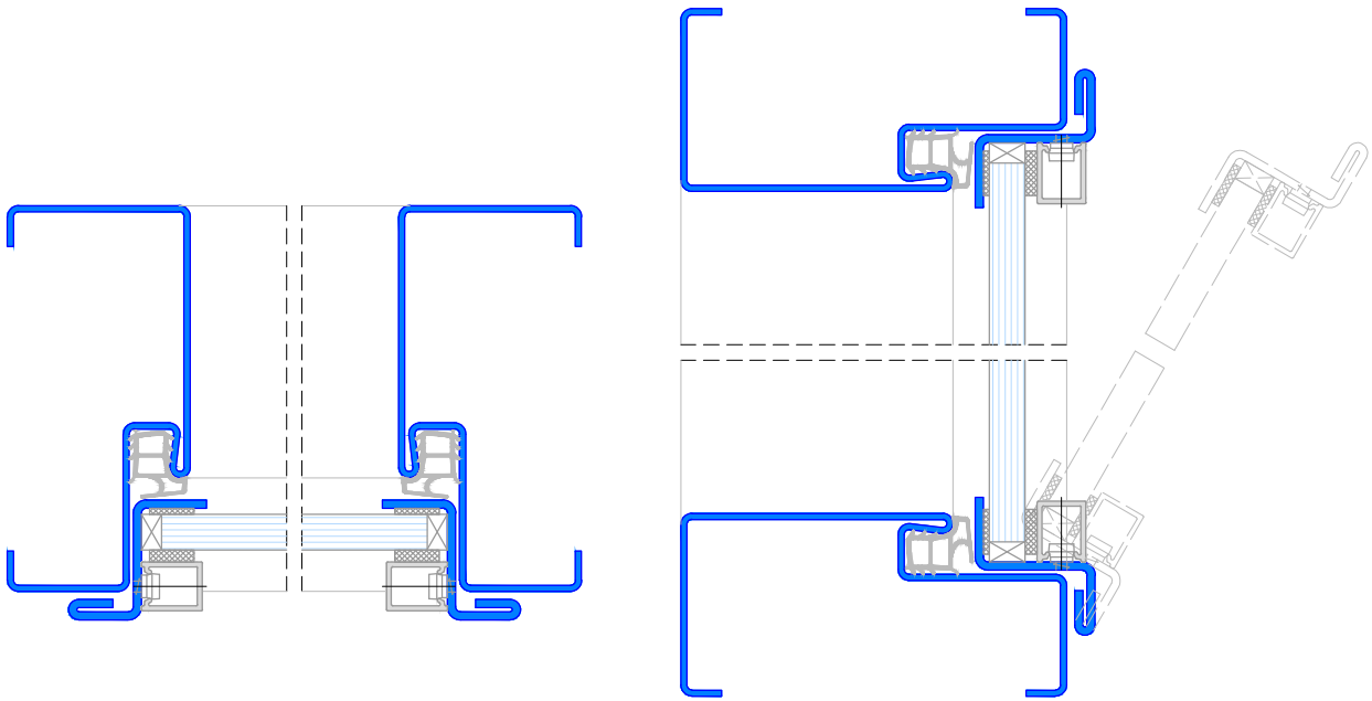
Fensterzarge einschalig
