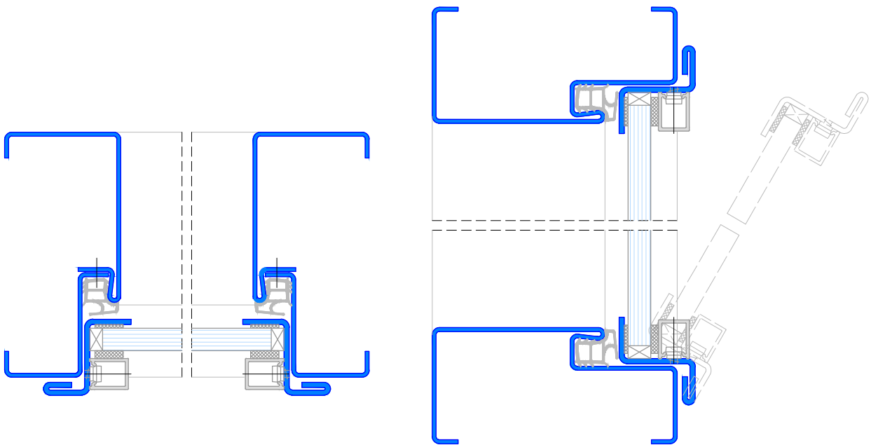
Fensterzarge zweischalig
