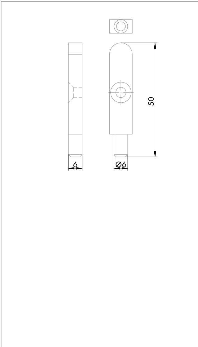
Standard-Auflagelasche
