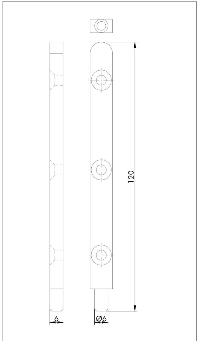
Sonder-Auflagelasche
