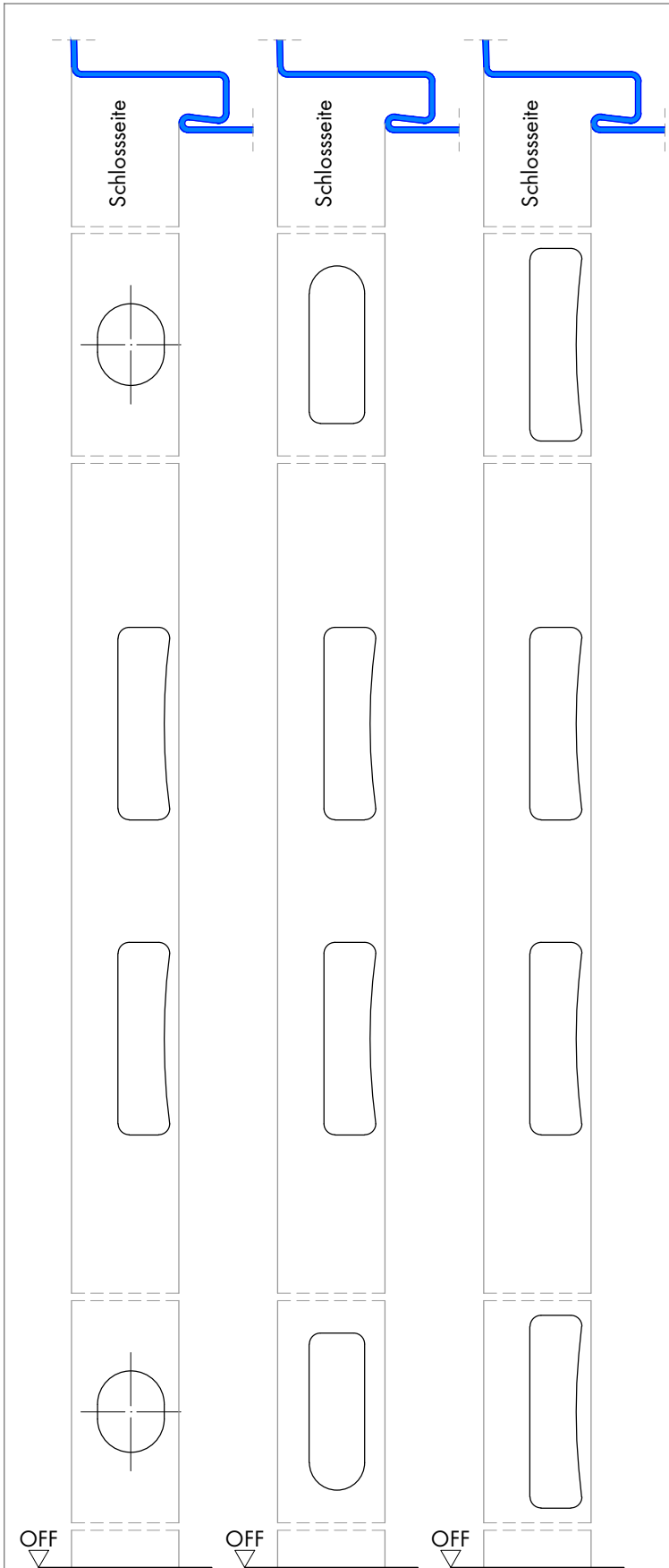
Dreifachverriegelung Variante und Maße auftragsbezogen
