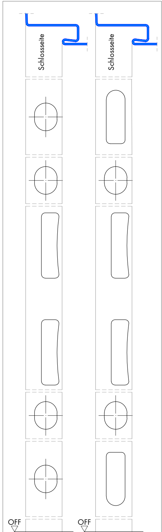
Mehrfachverriegelung Variante und Maße auftragsbezogen
