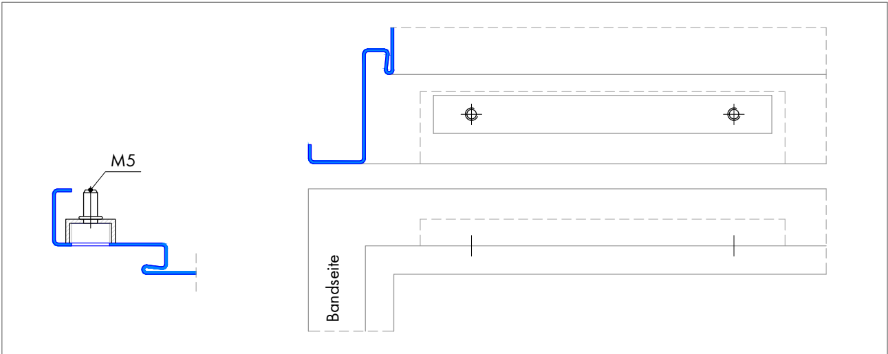
ITS mit Gleitschiene Montage im Kopfteil
