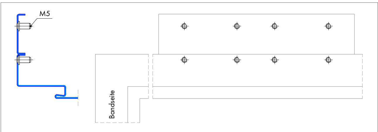
Drehflügelantrieb Kopfmontage Bandseite
