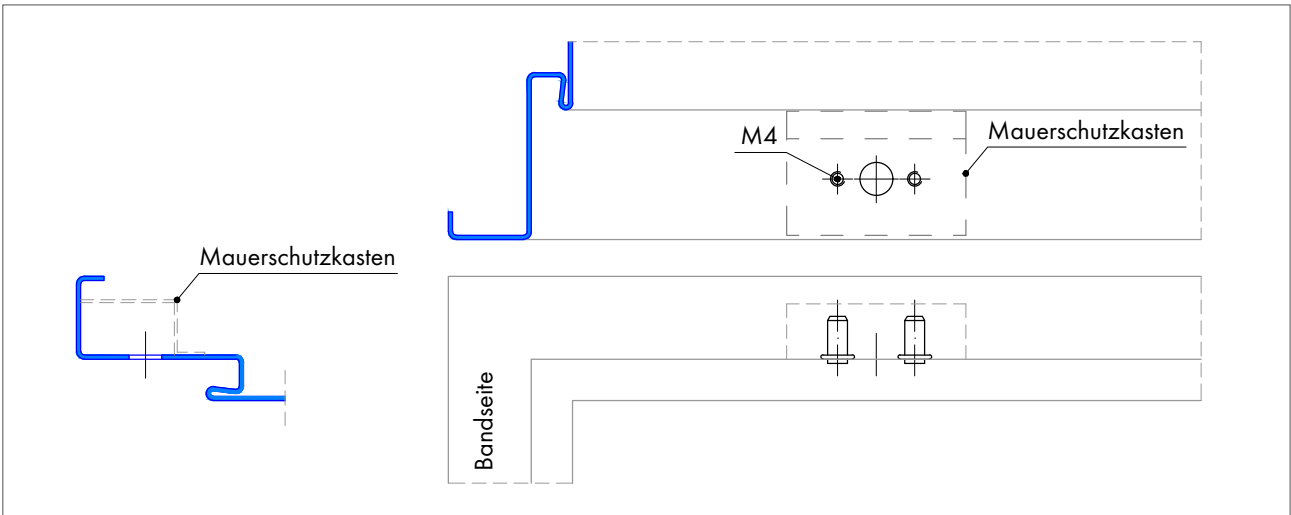
Türöffnungsbegrenzer Montage im Kopfteil
