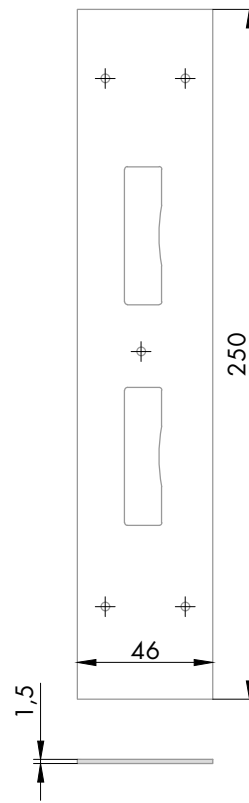
aufgesetztes Edelstahlschließblech stumpfe Ausführung
