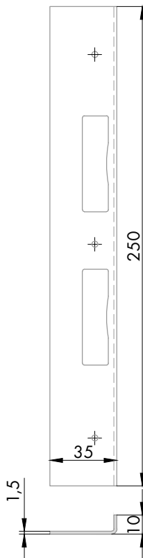
aufgesetztes Edelstahlschließblech gefälzte Ausführung
