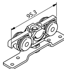
3 Rollapparat
