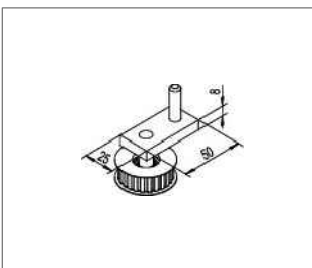
Synchronbeschlag
