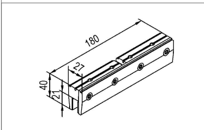
4 Glasklemmstück
