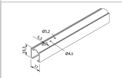
1 Laufschiene
