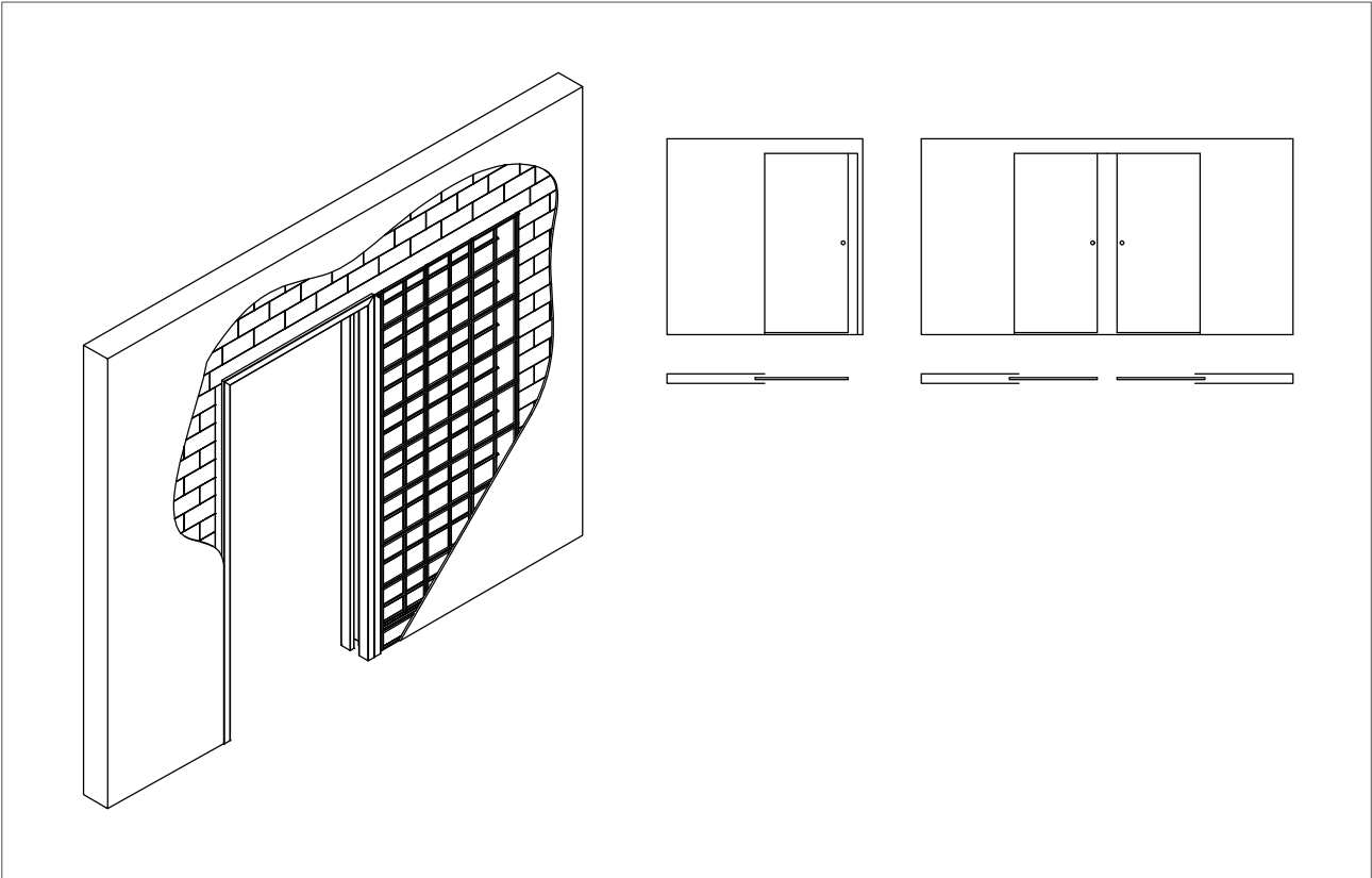
Einlaufkasten für Mauerwerkswände
