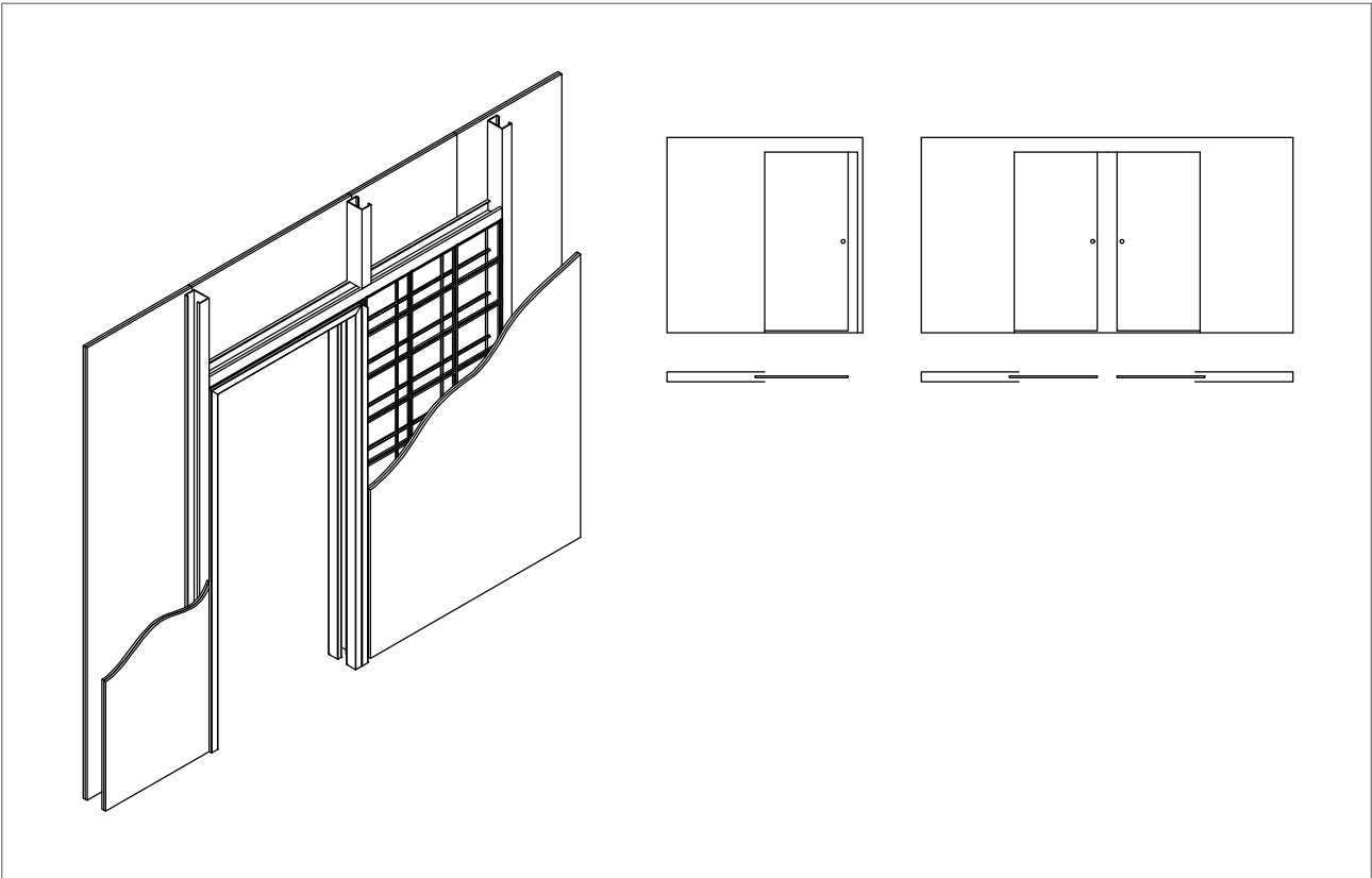
Einlaufkasten für Ständerwerkswände
