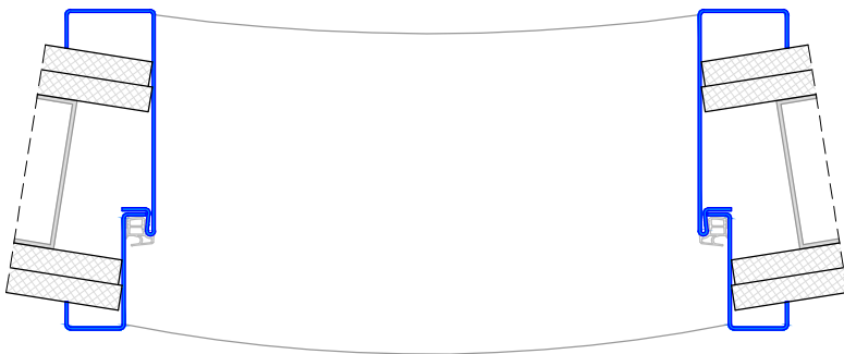
Schnitt A-A
