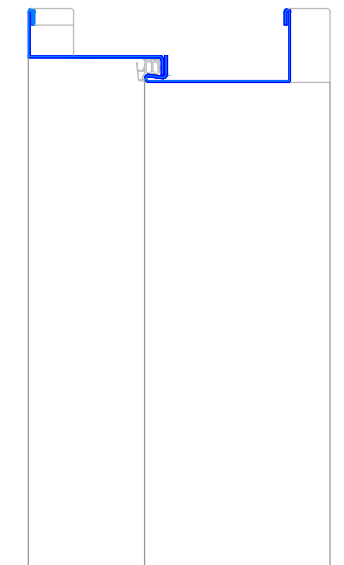
Schnitt B-B
