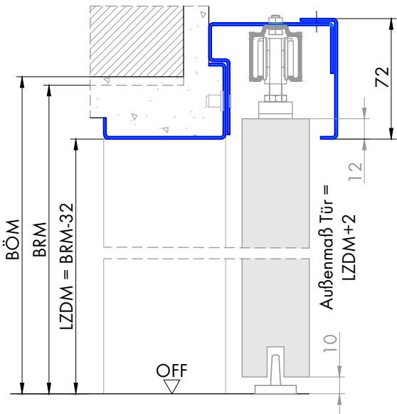
Schnitt B-B
