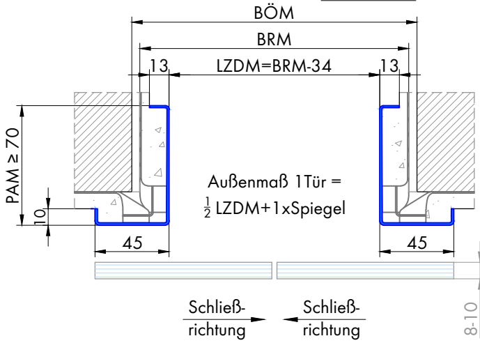
Schnitt A-A
