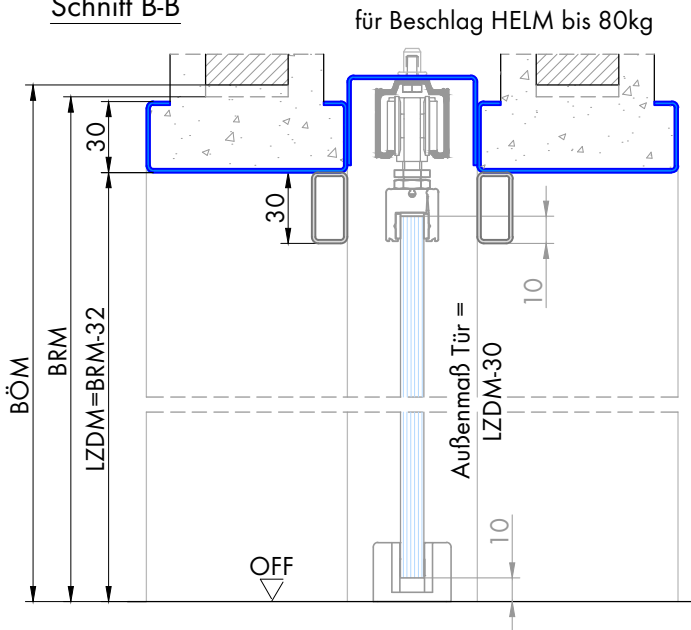
Schnitt B-B
