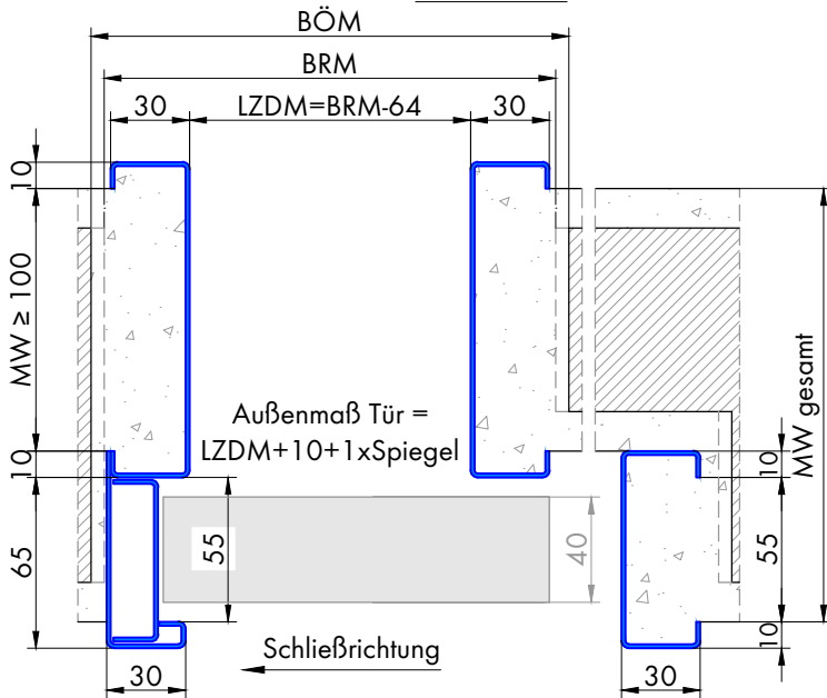
Schnitt A-A
