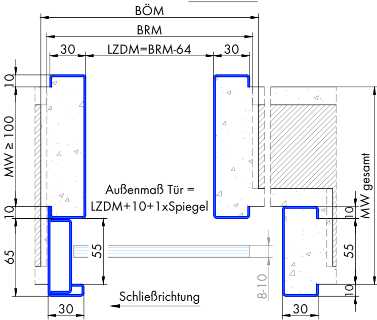
Schnitt A-A
