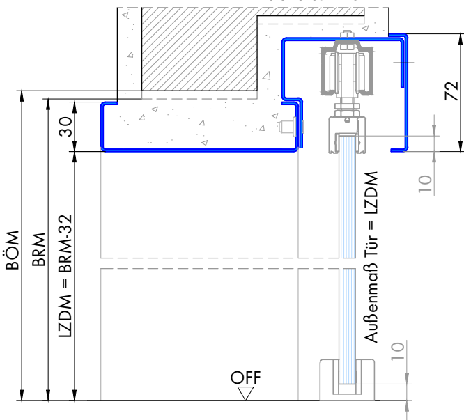
Schnitt B-B
