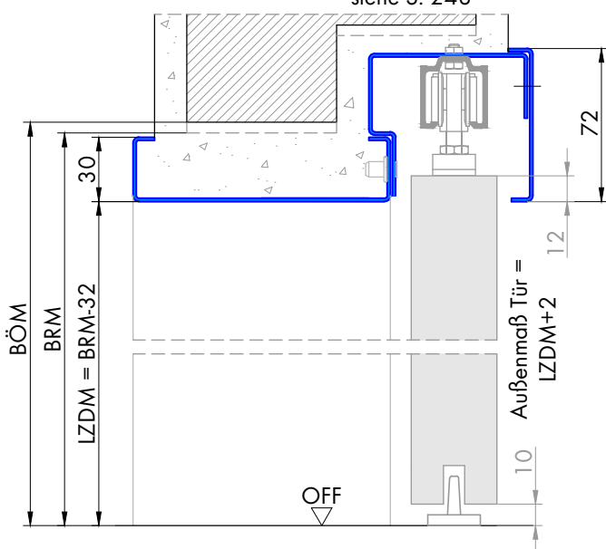
Schnitt B-B
