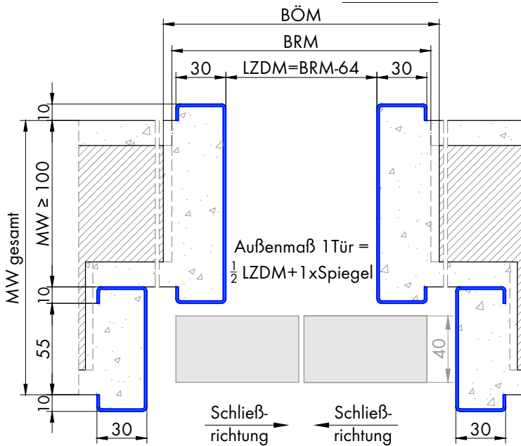
Schnitt A-A
