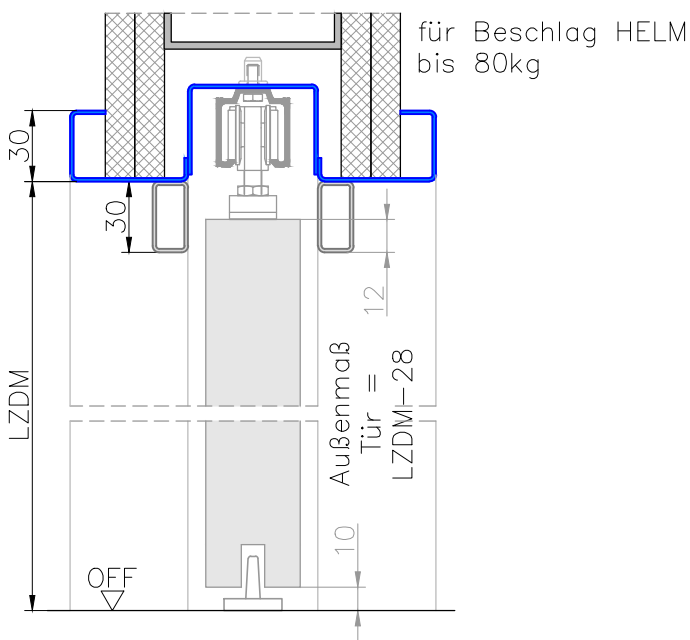
Schnitt B-B
