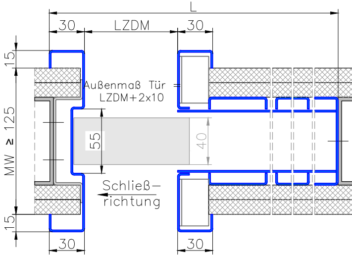
Schnitt A-A
