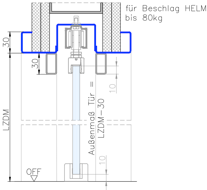
Schnitt B-B
