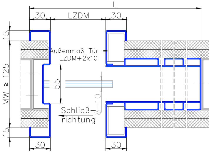
Schnitt A-A
