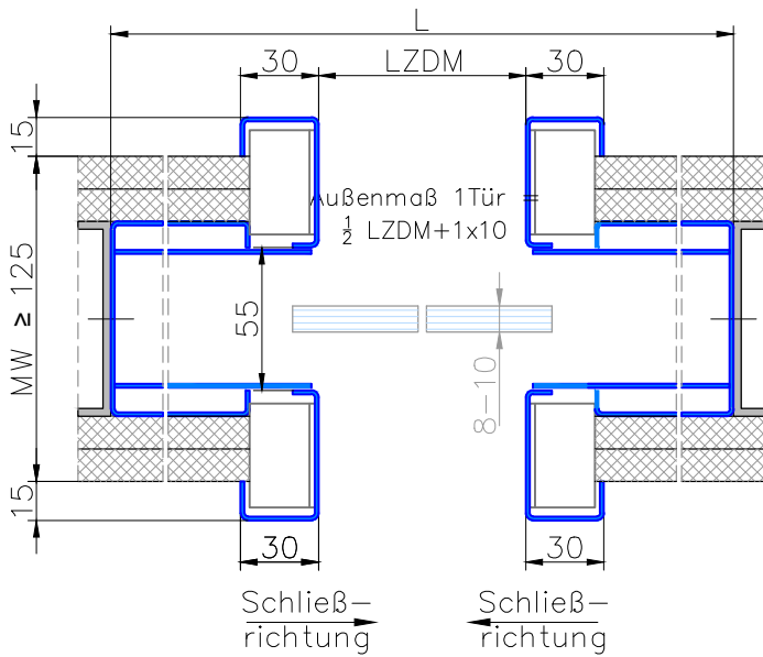
Schnitt A-A
