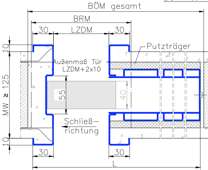
Schnitt A-A
