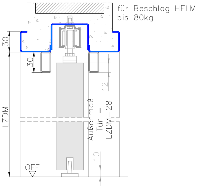
Schnitt B-B
