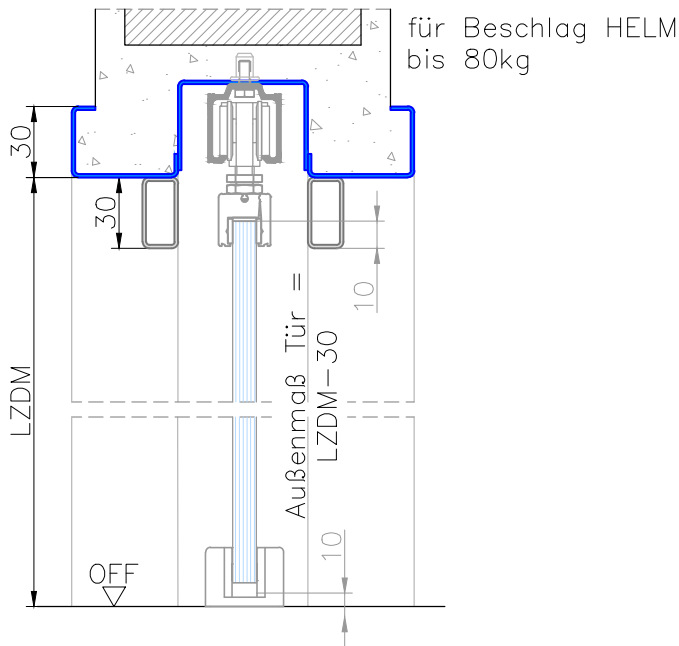
Schnitt B-B
