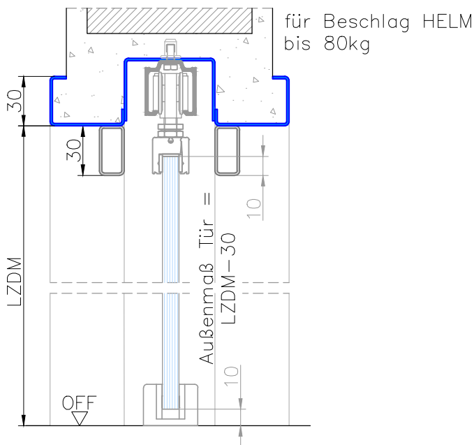
Schnitt B-B
