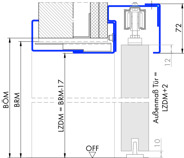
Schnitt B-B
