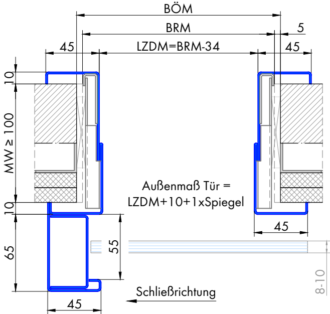
Schnitt A-A
