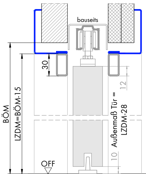
Schnitt B-B
