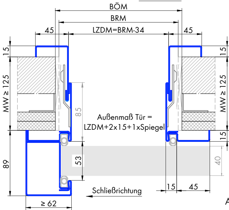
Schnitt A-A
