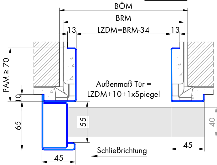
Schnitt A-A
