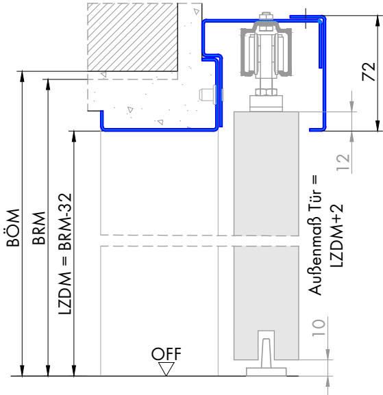
Schnitt B-B
